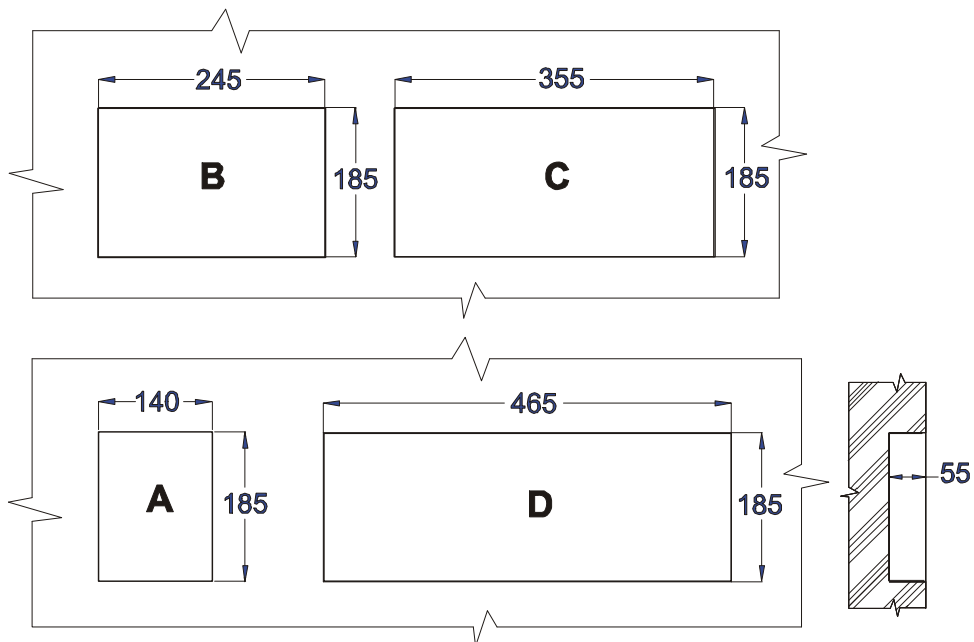
Obr. 1 Odporúčané montážne otvory v stene podľa typu EV Doporučené montážní otvory ve stěně podle typu EV
